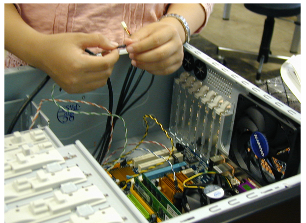
3. 配線中
